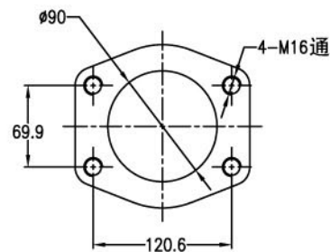
法兰 Flange SAE 3-1/2"
